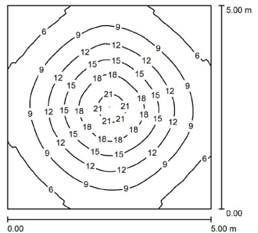
Gráfico de distribuição de luz - Isolux SL 3 - Para altura de 3 metros Led Oslon LED 120°
